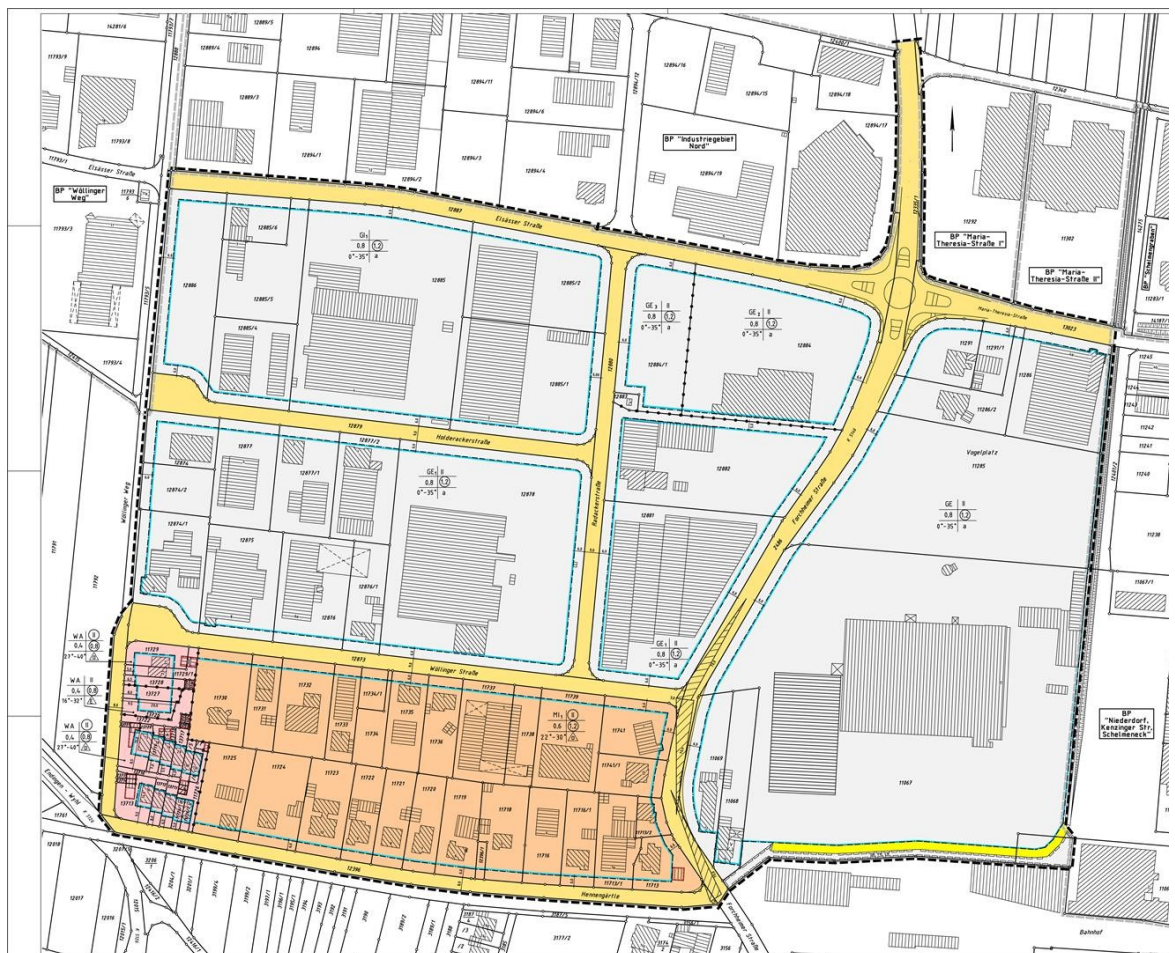
Rechtskräftiger B-Plan (unmaßstäblich)
